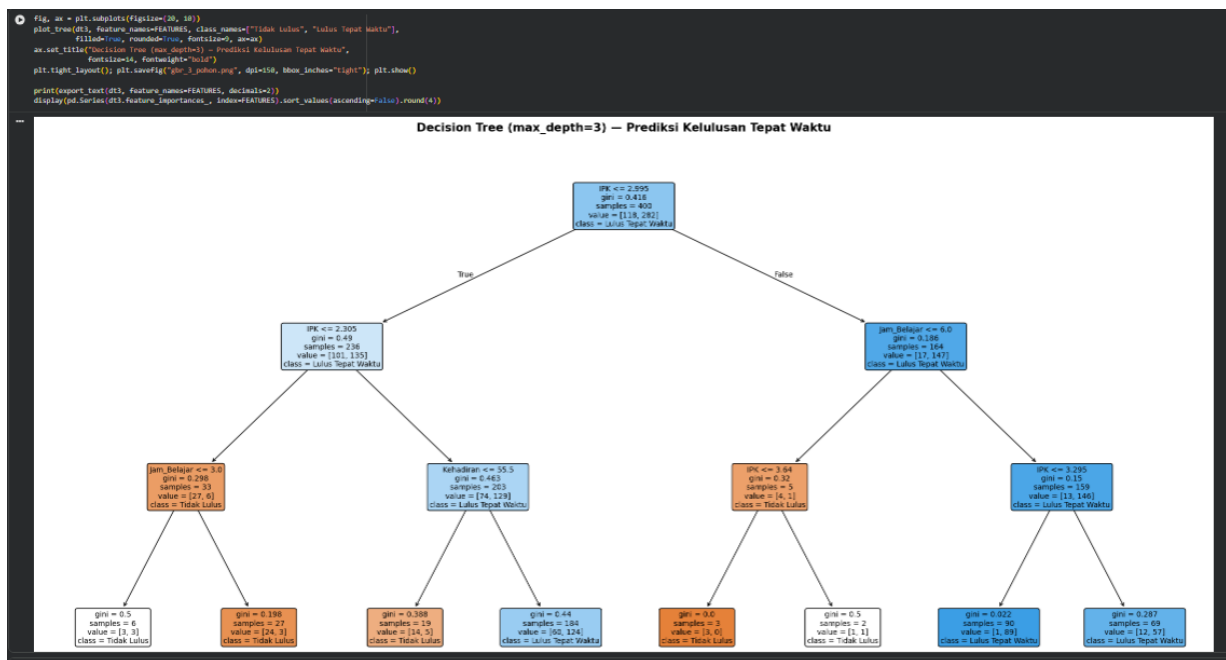
Gambar 6. Visualisasi pohon keputusan dengan max_depth=3
