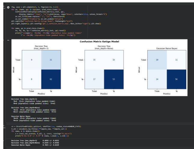
Gambar 5. Confusion matrix dan validasi silang lima lipatan
