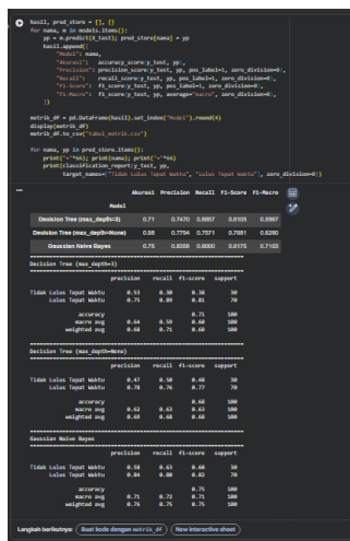
Gambar 4. Metrik evaluasi dan classification report
